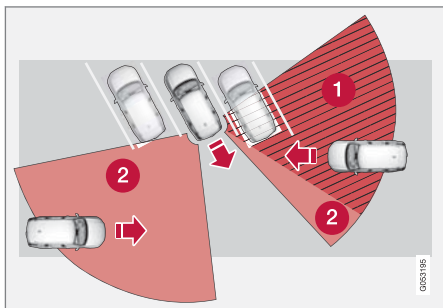
비좁은 주차 공간에서는 CTA가 한쪽 방향을 전혀 볼 수 없을 수 있습니다.
