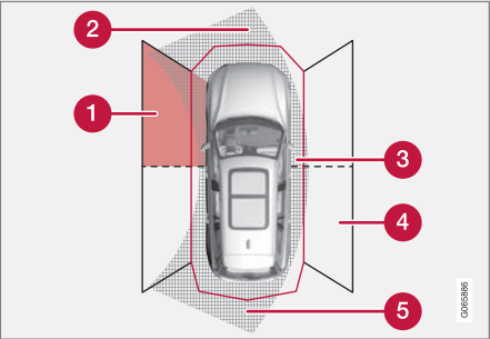
물체를 탐지할 수 있는 주차 센서 구역.
