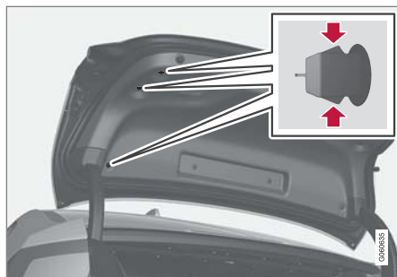
패널 고정 클립.
