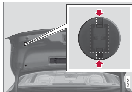
클립의 직사각형 부분을 차량의 세로 방향으로 맞춥니다.
