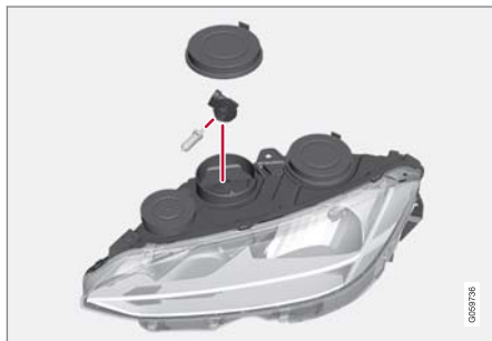
좌측 전조등.
