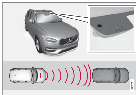
레이더 유닛 80 의 위치.
