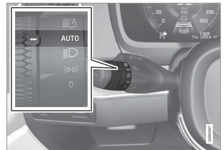
AUTO 위치에 있는 레버 스위치 회전 링.
