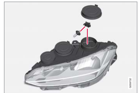
좌측 전조등.
