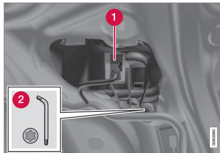
우측의 램프 하우징과 커버.
