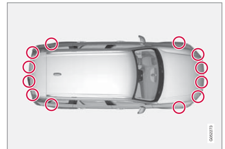
주차 센서 위치 137 .
