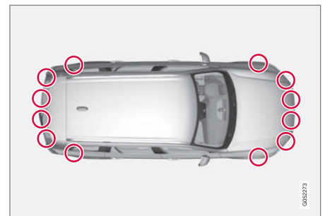
주차 센서 위치 123 .
