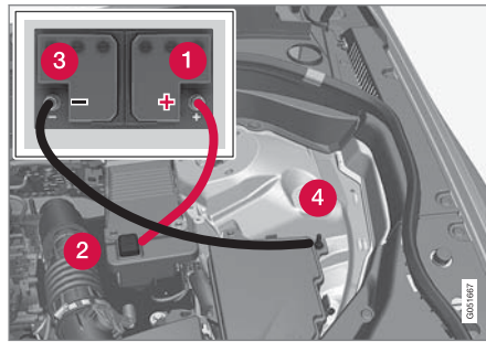
점프 시동 지점.
