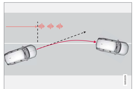
차선유지 지원 시스템은 스티어링 휠 진동을 통해 경보를 제공합니다. 115
